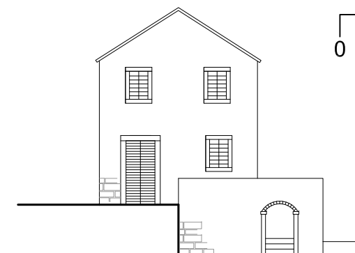
ISTOČNA FASADA
