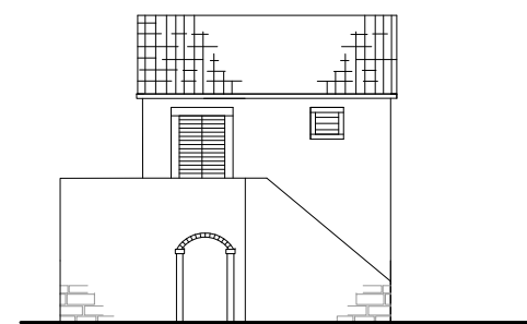
ZAPADNA FASADA
