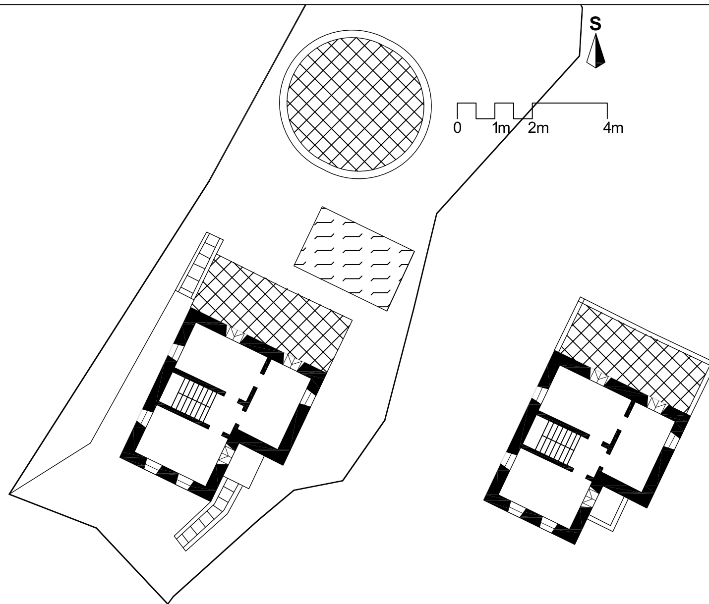
OSNOVA SPRATA
