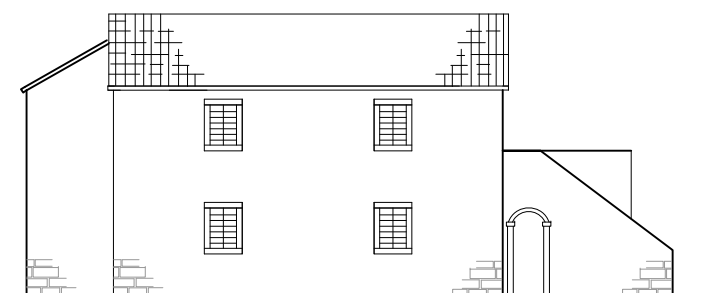
ISTOČNA FASADA
