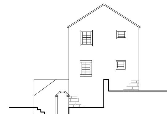
ZAPADNA FASADA
