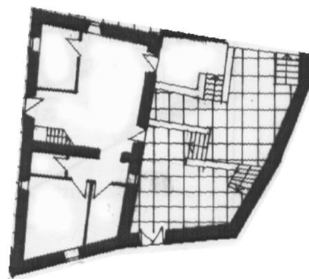
OSNOVA PRIZEMLJA
