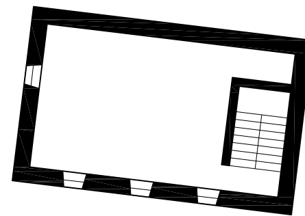
OSNOVA SPRATA objekat 1
