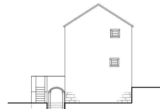
ZAPADNA FASADA
