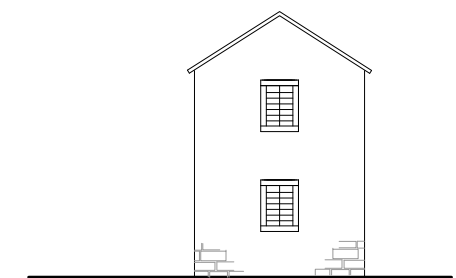
SJEVEROZAPADNA FASADA
