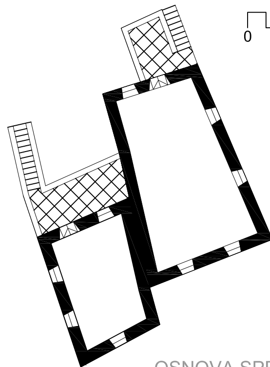
OSNOVA SPRATA
