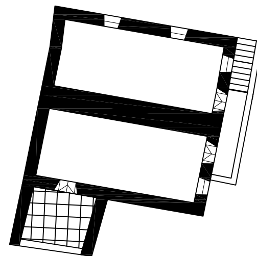
OSNOVA SPRATA
