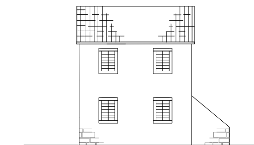
JUGOZAPADNA FASADA
