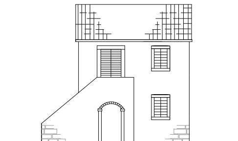
SJEVEROISTOČNA FASADA
