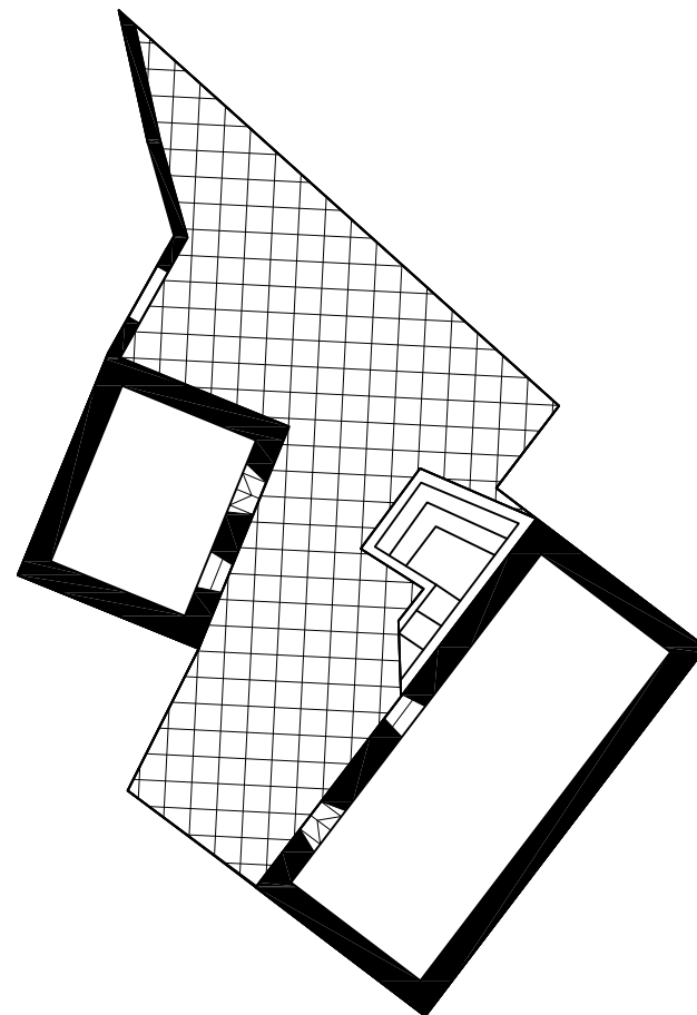
OSNOVA PRIZEMLJA
