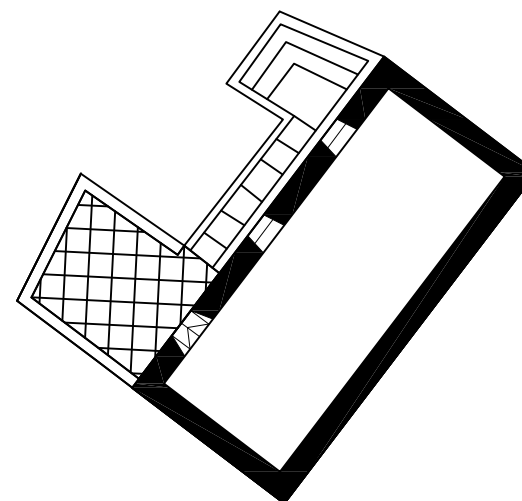
OSNOVA SPRATA
