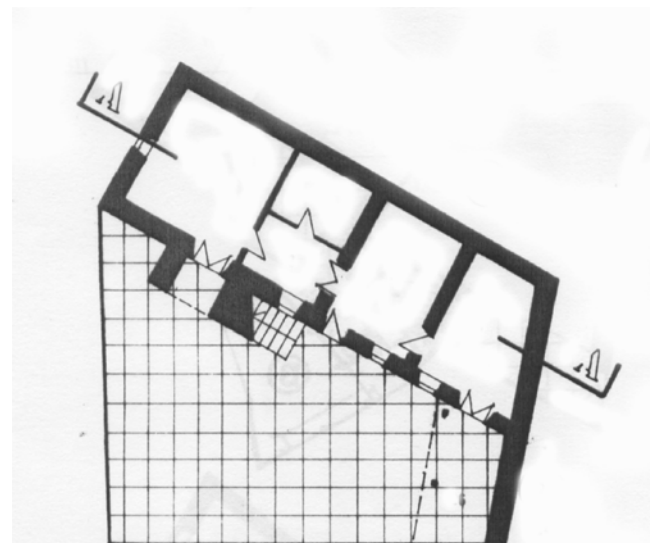
OSNOVA PRIZEMLJA
