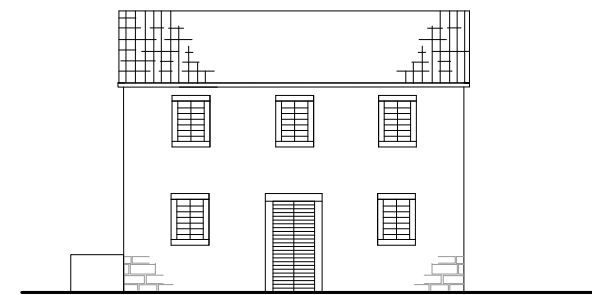
ZAPADNA FASADA
