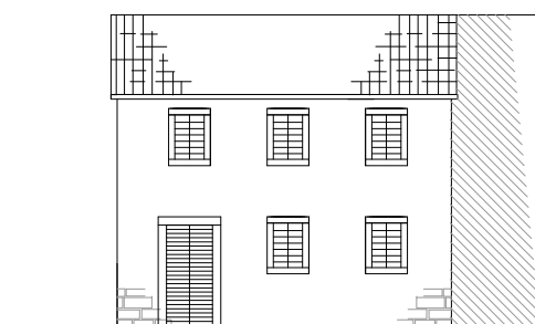
SJEVERNA FASADA
