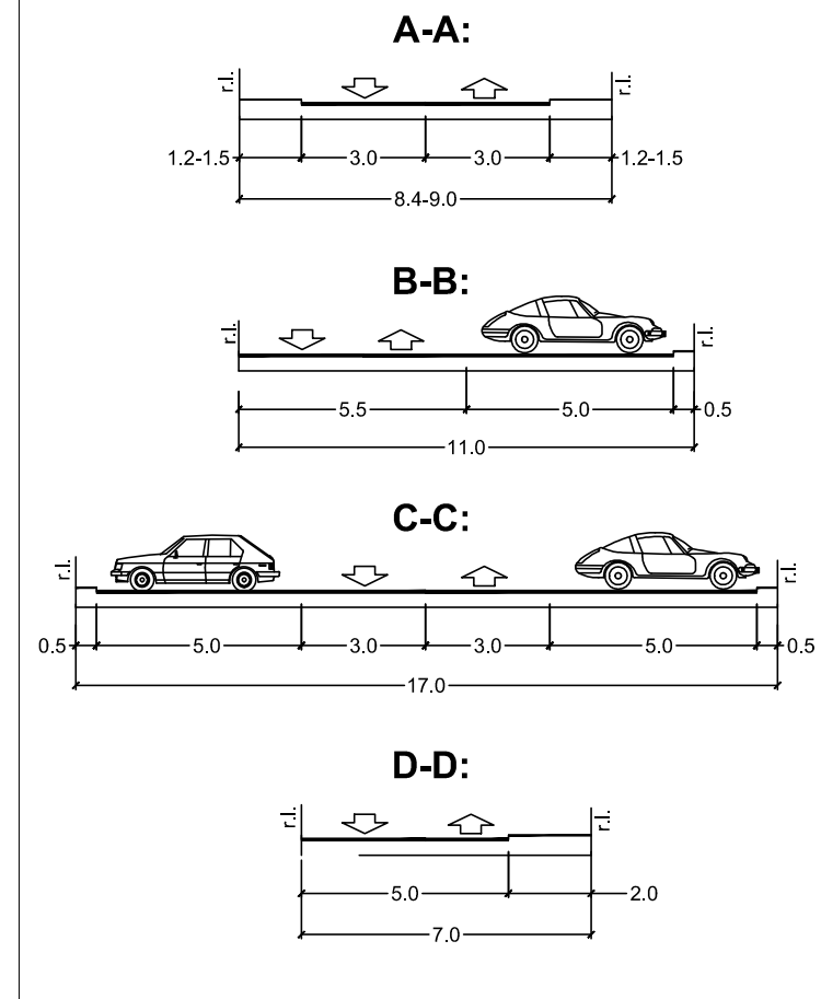
Poprečni profili, R = 1:200
