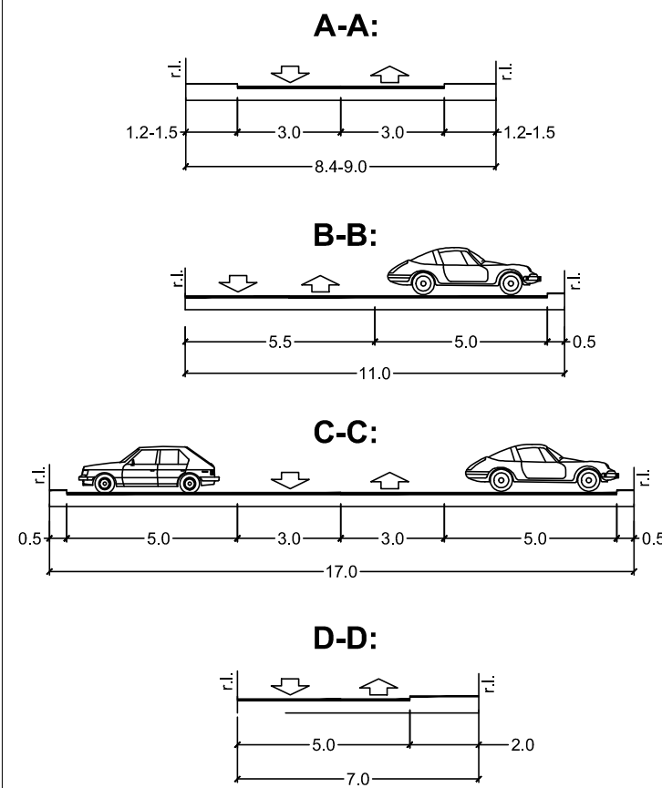
Poprečni profili, R = 1:200
