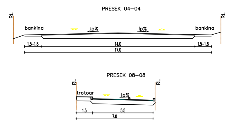
POPREČNI PROFILI SAOBRAĆAJNICA R 1:200
